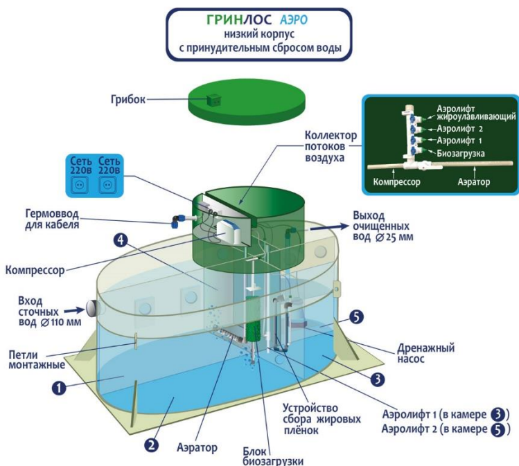
Рисунок 2. Схема модели с принудительным сбросом сточных вод и низким корпусом
