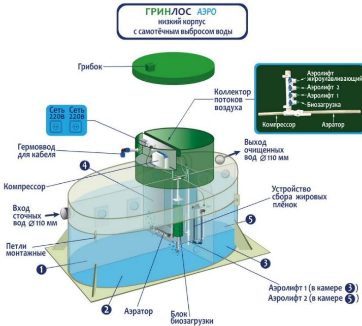
Рисунок 1. Схема модели с самотечным сбросом сточных вод и низким корпусом
